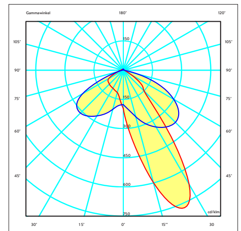
Lichtverteilungskurve DIAMANT FIT5 E-Line 30-72 W, 25° asymmetrisch rechts oder links light emitting diag. DIAMANT FIT5 E-Line 30-72W, 25° asymmetrical right and left
